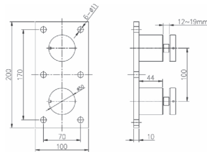
Kahe Noktasal Cam Tutucu
