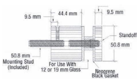
Kahe Ayarlı Noktasal Cam Tutucu Kahe Adjustable Point Glass Holder
