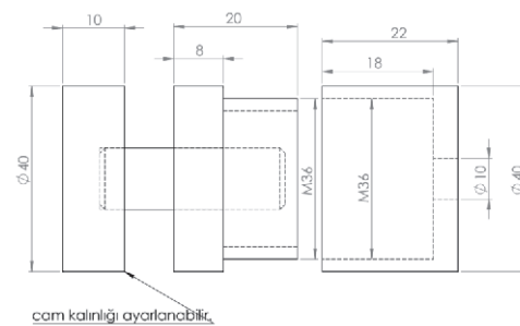
Kahe Ayarlı Noktasal Cam Tutucu Kahe Adjustable Point Glass Holder
