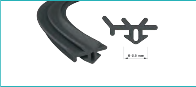
Tırnaklı Çakma 6-6,5 mm. Spiked Nailing 6-6,5 mm.
