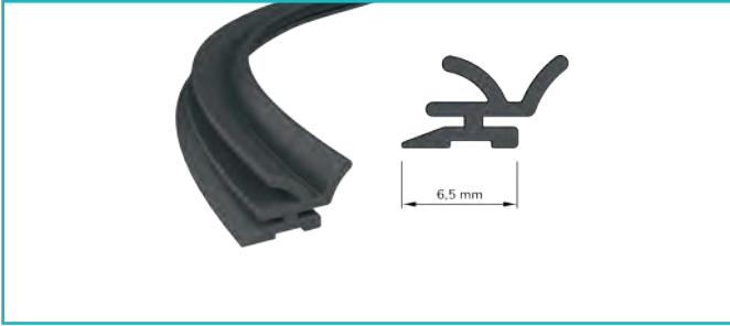
Yeni Aldoks Çift kulak 6,5 mm. New Aldoks Double Ear 6,5 mm.
