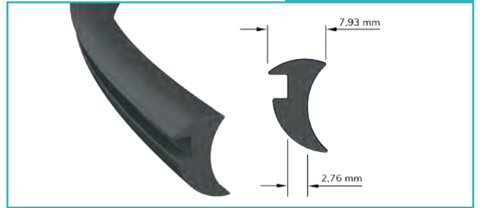
İç Cam Contası Interior Glass Joints
