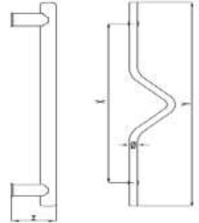
AYNALI BORU ÇEKME D KOL PULL HANDLE مسكة أبواب زجاج CODE : AB 172-O
