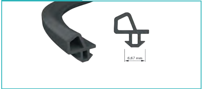
Plastik Doğrama Contası Plastic Joinery Joint
