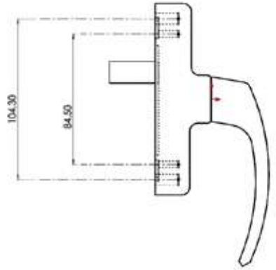
ISPANYOLET KOL CREMONE HANDLE
