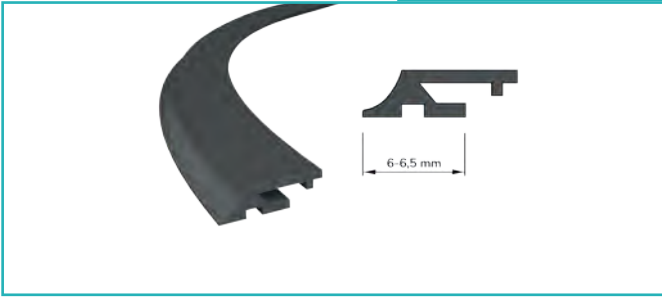
Yeni Maçalı 6-6,5 mm. New Cord Seal 6-6,5 mm.
