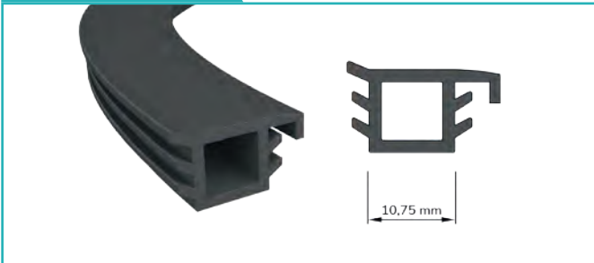
Çelik Kapı Fitili Steel Door Seal
