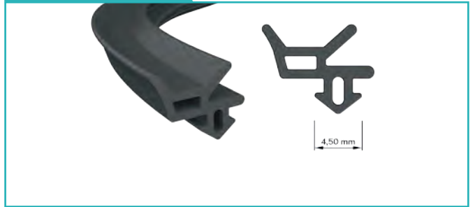
Plastik Doğrama Contası Plastic Joinery Joint
