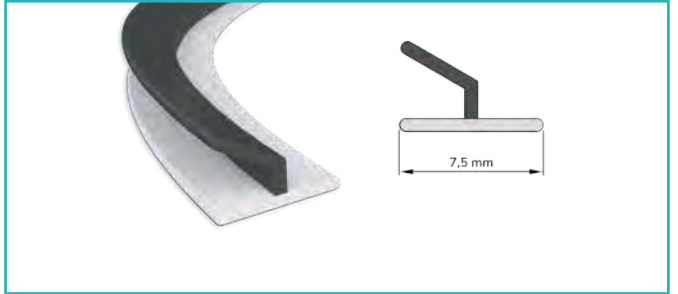
Sert Yumuşak Aldoks 7,5 mm. Hard Soft Aldoks 7,5 mm.
