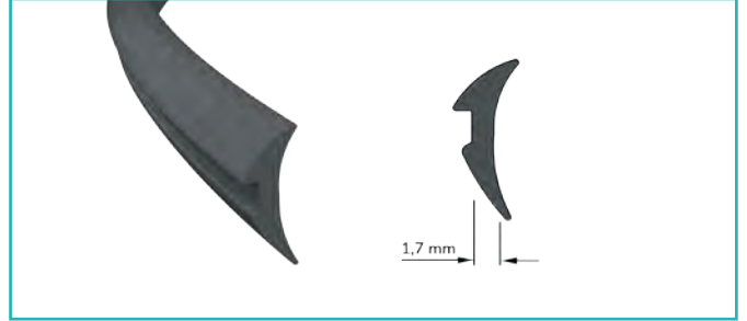
İç Cam Contası 1,7 mm. Interior Glass Joints 1,7 mm.
