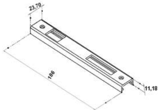
KAPI KİLİT KARŞILIĞI STRIKER FOR DOOR اكسسوارات أبواب CODE : AB 091-EK
