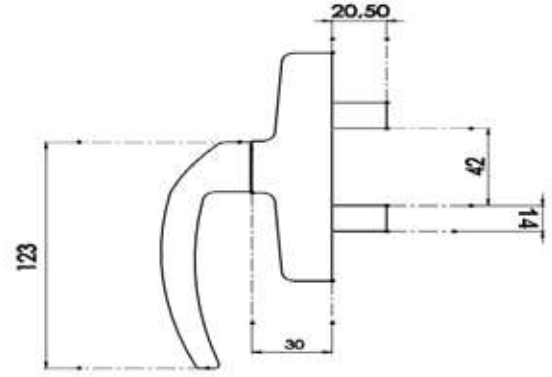
EKSENEL KOL SAÇ TEK MAÇA WINDOW HANDLE
