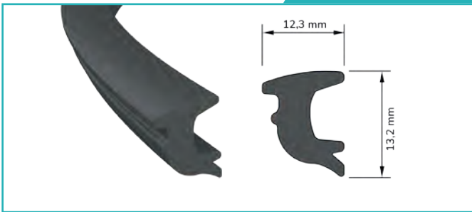
Isı Cam Contası Heating Glass Joints
