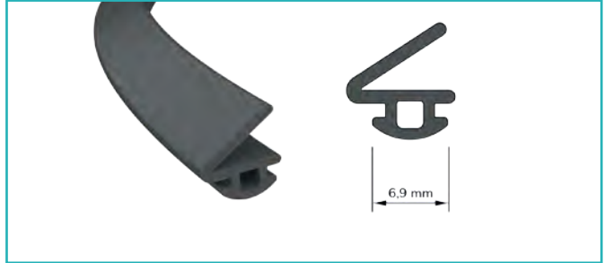
Kasa Kanat Contası Casing Wing Joint
