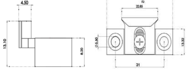
AYARLI İSPANYOLET KARŞILIĞI SETRİSKURLU ADJUSTUBLE STRIKER
