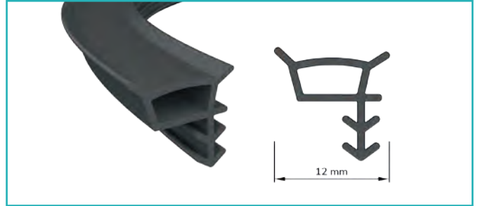
Ahşap Doğrama Fitili Wood Work Seal
