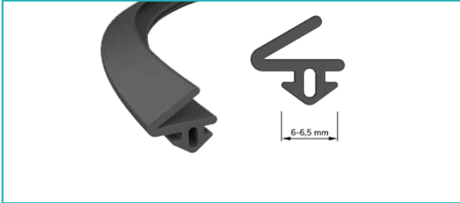
Yarık Conta 6-6,5 mm. Splint Joint 6-6,5 mm.
