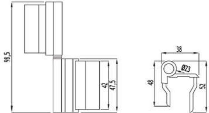
C 60 KAPI GEÇME MENTEŞE DOOR HINGE
