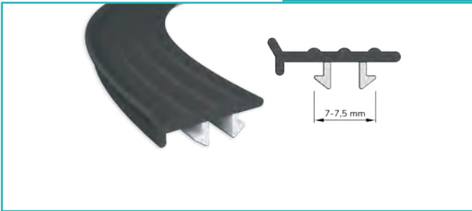
Sert Yumuşak Çakma Maçalı 7-7,5 mm. Hard Soft Nailing Cored 7-7,5 mm.
