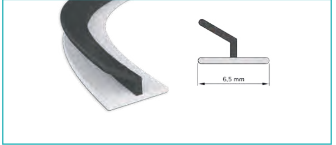
Sert Yumuşak Aldoks 6,5 mm. Hard Soft Aldoks 6,5 mm.
