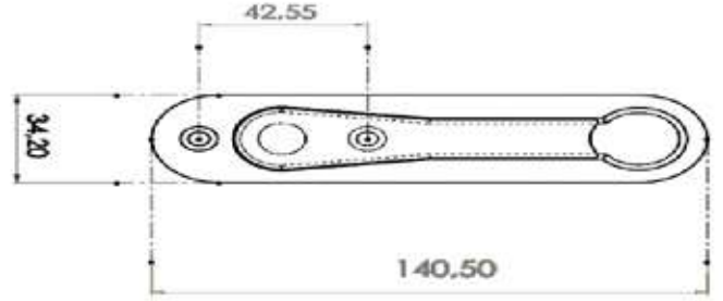
TETİK KOL SLIDING HANDLE
