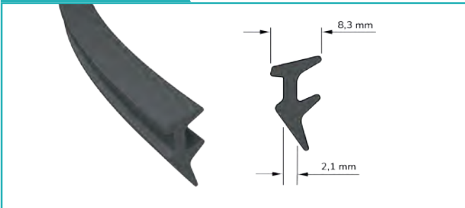
İç Cam Contası Interior Glass Joints
