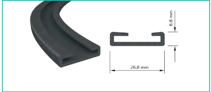
Sac Kenar Fitili Sheet Metal Edge Seal
