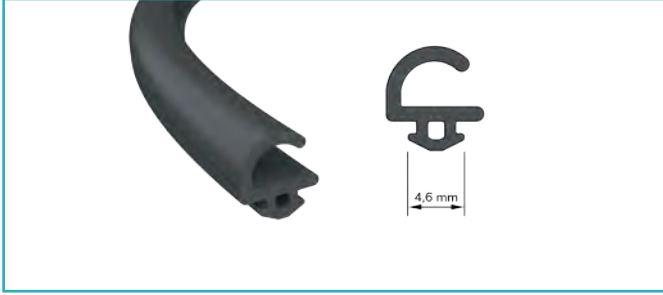
Yark Kanat Contası Cleft Wing Seal
