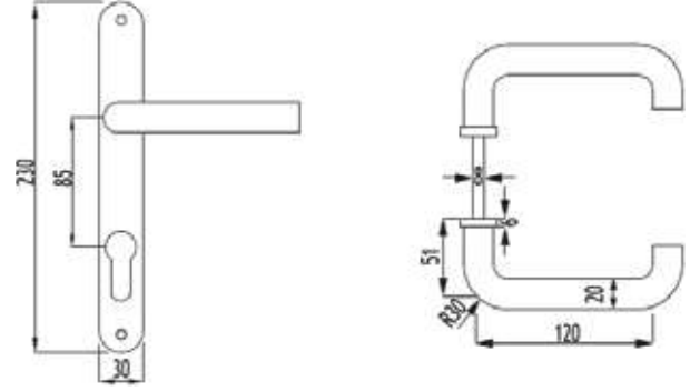
YARIM AY KOL PULL HANDLE
