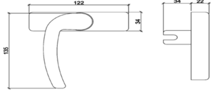
CEPHE KOL KIVRIK ZAMAK ÇİFT MAÇA FACADE WINDOW HANDLE
