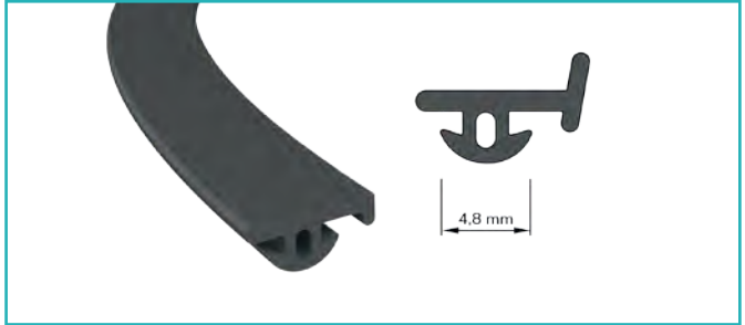
Kanat Contası Rope Joints
