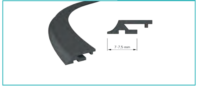
Yeni Maçalı 7-7,5 mm. New Cord Seal 7-7,5 mm.
