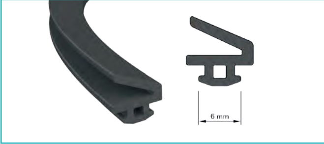
Yarı Kanat Contası Cleft Wing Seal
