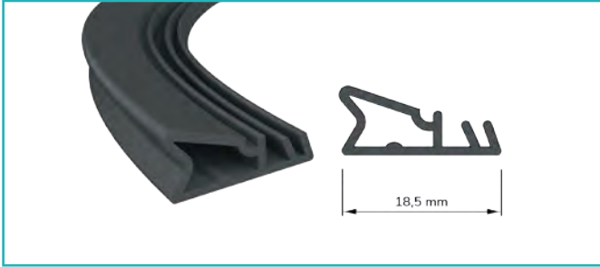
Ahşap Doğrama Fiteli Wood Work Seal
