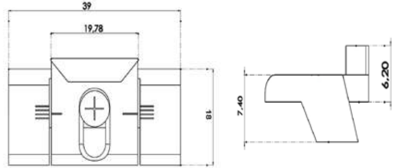
SİSTEM SERİ CEPHE KARŞILIĞI ADJUSTUBLE STRIKER 1
