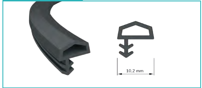
Ahşap Doğrama Fitili Wood Work Seal
