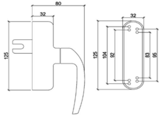
EKSENEL KOL SAÇ TEK MAÇA WINDOW HANDLE
