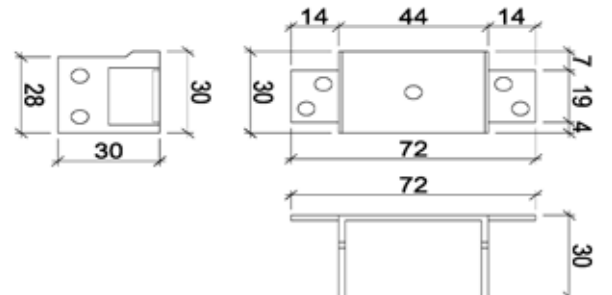
PVC ORTA KAYIT BAĞLANTI TAKOZU PVC STEEL MIDDLE JOINT مثبت بروفيلات ألومنيوم CODE : AB 012-F
