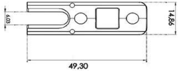
CEPHE KARŞILIK YÜKSELTİCİ ADJUSTUBLE STRIKER
