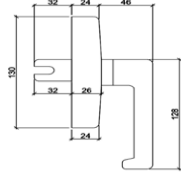
EKSENEL KOL ZAMAK TEK MAÇA WINDOW HANDLE
