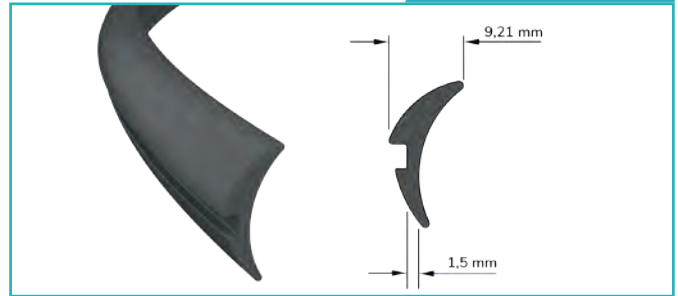
İç Cam Contası Interior Glass Joints
