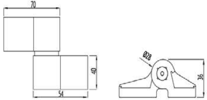
C 60 KAPI MENTEŞE KÖŞELİ DOOR HINGE
