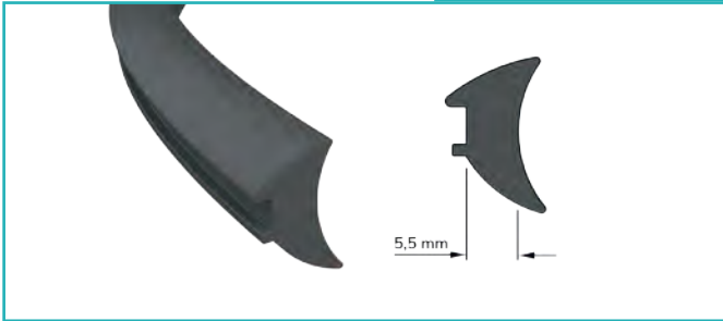
İç Cam Contası 5,5 mm. Interior Glass Joints 5,5 mm.
