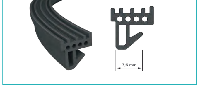
Isı Yalıtım Fitolu Thermal Insulation Seal
