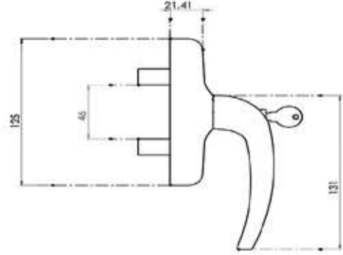
EKSENEL KOL SAÇ TEK MAÇA CREMONE HANDLE WITH KEY
