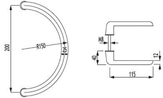
YARIM AY KOL VİDALI PULL HANDLE
