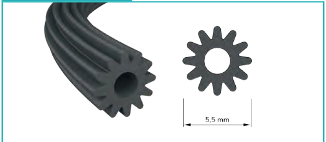
Sineklik Gerğı Kordonu Fly Net Cordon
