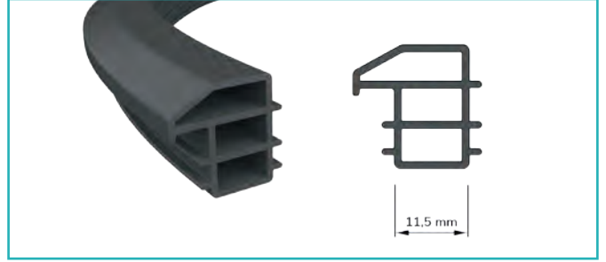
Çelik Kapı Fitili Steel Door Seal
