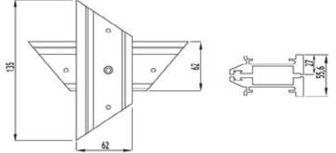
ASAŞ KAPI MENTEŞE WINDOW HINGE FOR DOOR
