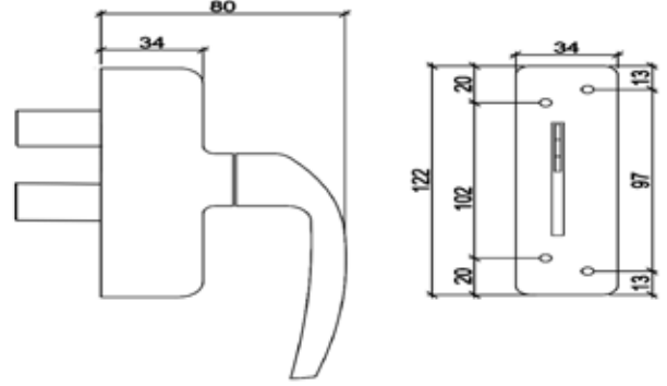
EKSENEL KOL ZAMAK İNCE TEK MAÇA WINDOW HANDLE
