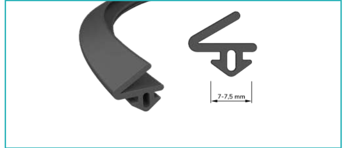
Yarık Conta 7-7,5 mm. Splint Joint 7-7,5 mm.
