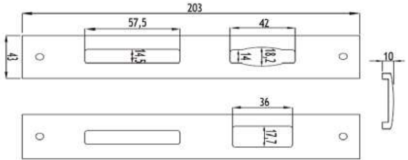
C 60 MAKARALI KİLİT KARŞILIĞI STRIKER FOR DOOR
