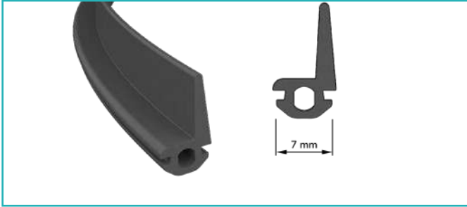
Isı Yalıtım Fiteli Thermal Insulation Seal
