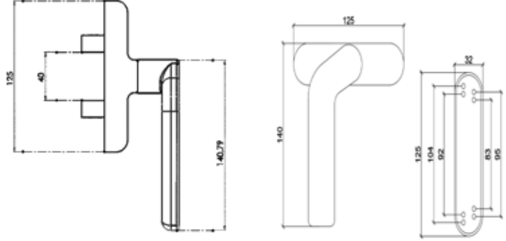
CEPHE KOL KIVRIK ZAMAK TEK MAÇA FACADE WINDOW HANDLE
