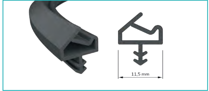
Ahşap Doğrama Fiteli Wood Work Seal
