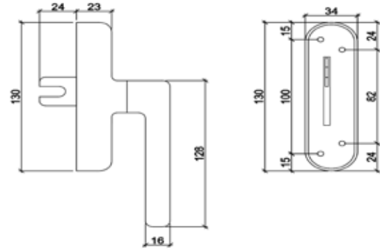
ELOKSAL EKSENEL KOL ZAMAK TEK MAÇA WINDOW HANDLE
