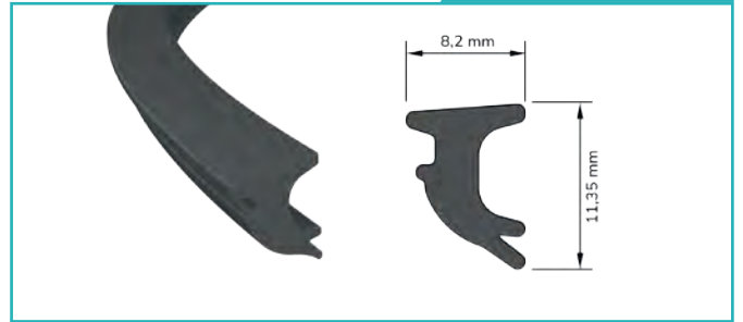
Isı Cam Contası Heating Glass Joints
