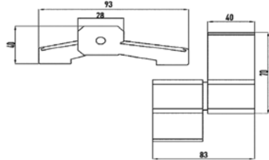
C 60 KAPI 3'LÜ MENTEŞE DOOR HINGE
