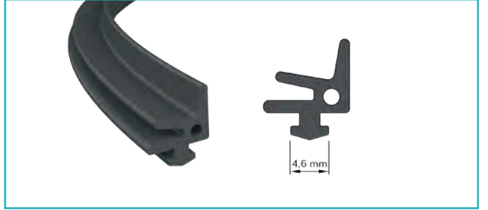
Kasa Kanat Contası Casing Wing Joint
