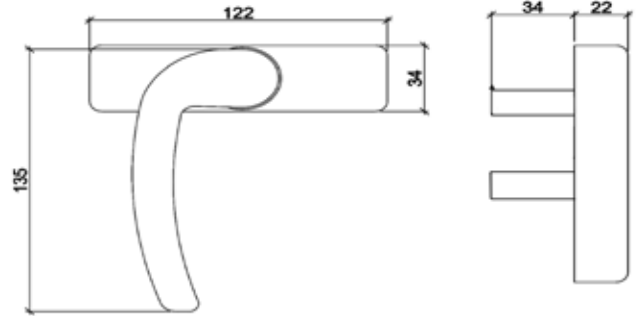
CEPHE KOL KIVRIK ZAMAK İNCE TEK MAÇA FACADE WINDOW HANDLE
