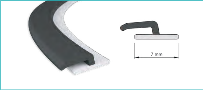
Sert Yumuşak Aldoks Hard Soft Aldoks
