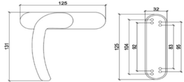
CEPHE KOL KIVRIK ZAMAK ÇİFT MAÇA FACADE WINDOW HANDLE
