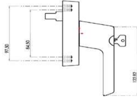
CEPHE KOL ZAMAK TEK MAÇA FACADE WINDOW HANDLE
