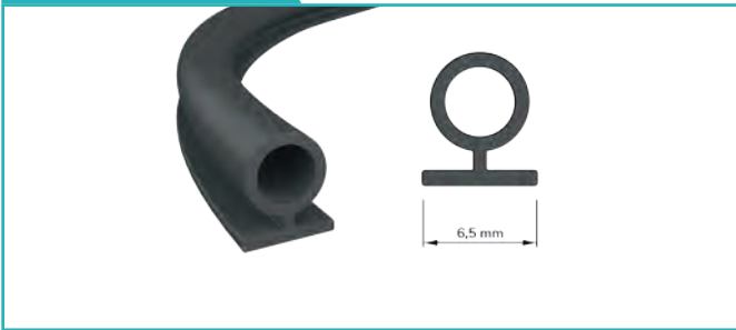
Omega Fitol 6,5 mm. Omega Seal 6,5 mm.
