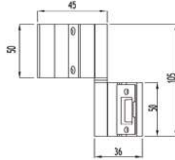
YUNAN MENTEŞE 3'LÜ WINDOW HINGE (EURO GROVE)
